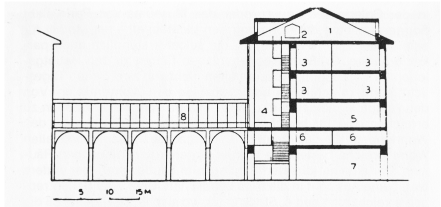
Abb. 6 Aufriß eines Phalanstères: 1. Dachgeschoß mit »camps cellulaire«, 2. Wassertanks, 3. Wohnungen, 4. Rue-Galerie, 5. Kommunikationsräume, 6. Mezzanin mit Wohnungen für Kinder, 7. Erdgeschoß mit Wagentdurchfahrten, 8. Rue-Galerie im 1. Stock mit Verbindung zwischen parallel liegenden Baukörpern. [nach BOLLEREY 1977]
